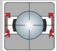
FUD UltraLife Dichtung
